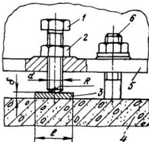
Рис. 2. Выверка оборудования с помощью регулировочных винтов:
