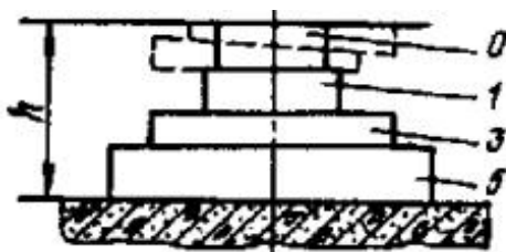
Рис. 6. Пирамидальный пакет подкладок:
