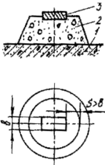
Рис. 8. Бетонная опора с металлической пластиной:
