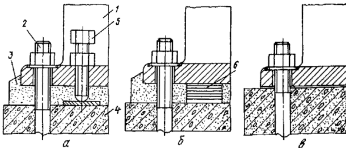
Рис. 1. Типы соединений "оборудование-фундамент":
