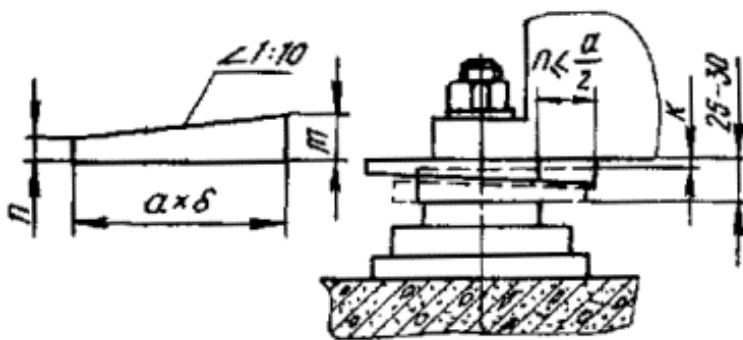
Рис. 7. Клиновые подкладки
