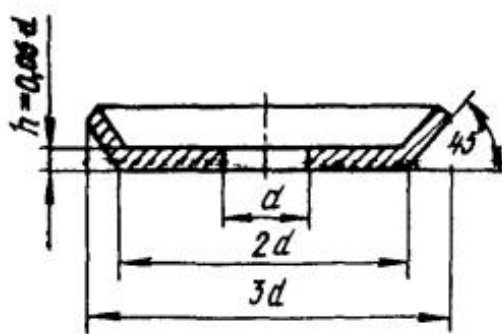
Рис. 1. Установочная шайба (наружный диаметр развертки шайбы 3,4 d ; материал - Ст3)
