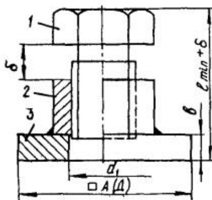
Рис. 2. Винтовая подкладка:
