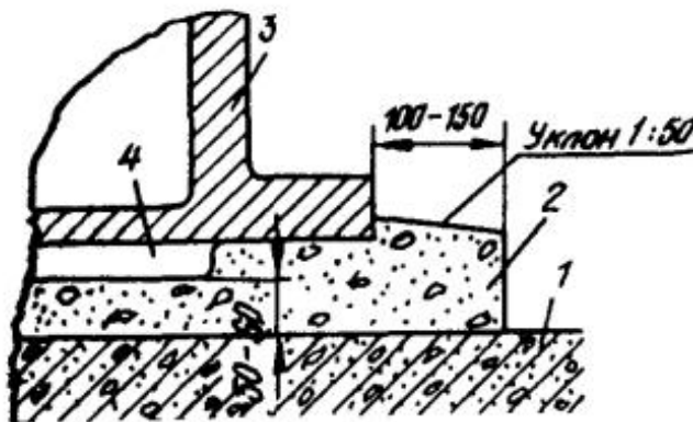
Рис. 9. Схема подливки оборудования:
