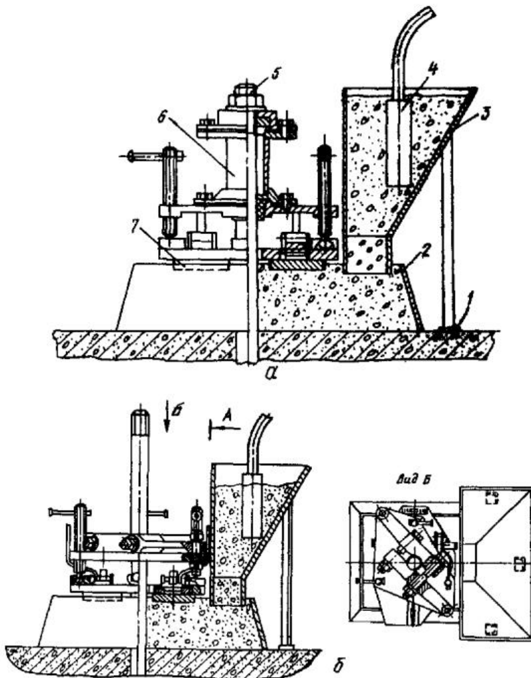
Устройство для установки опорных элементов на фундаменте:
