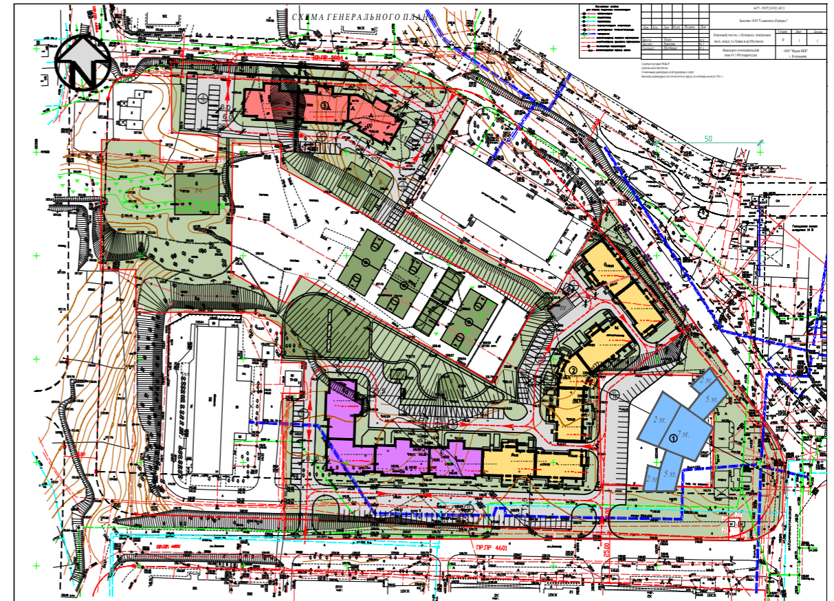
Схема генерального плана застройки микрорайона «Центр»
