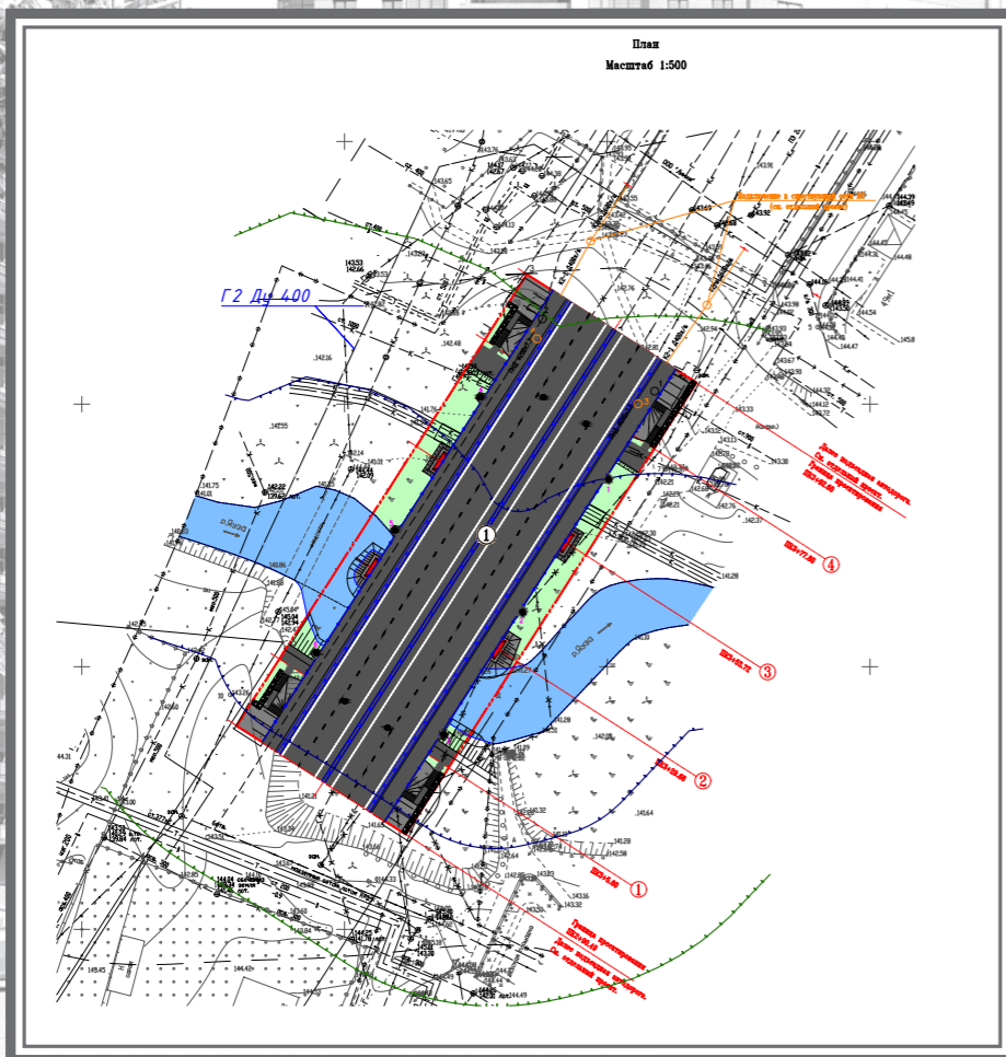
Генеральный план фрагмента. Мост.
